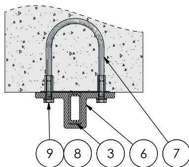
B-B
